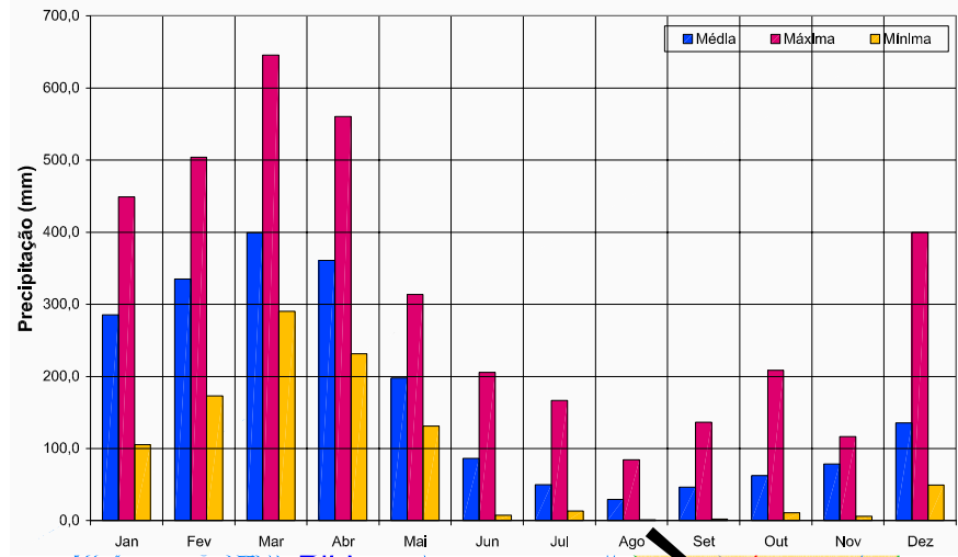
POSTO: BRASIL NOVO (ANA) VARIAÇÃO MENSAL DA PRECIPITAÇÃO PERÍODO: JAN/96 A DEZ/05
