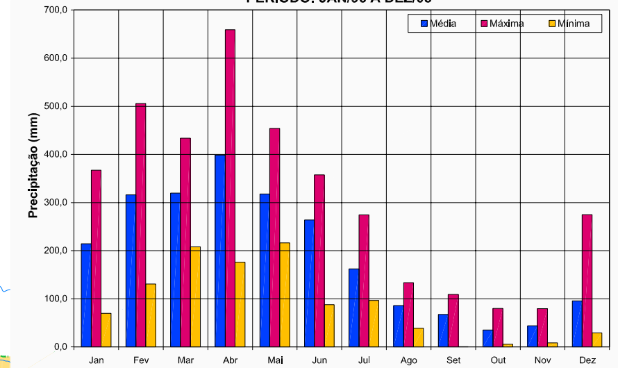
POSTO: P MOZ - (INMET) VARIAÇÃO MENSAL DA PRECIPITAÇÃO PERÍODO: JAN/96 A DEZ/05
