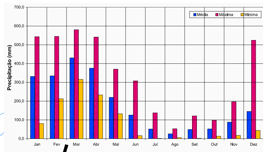
POSTO: ALTAMIRA (INMET) VARIAÇÃO MENSAL DA PRECIPITAÇÃO PERÍODO: JAN/96 A DEZ/05
