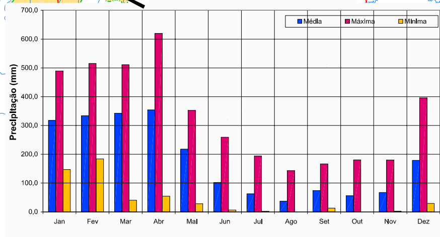
POSTO: FAZ. CIPAÚBA (ANA) VARIAÇÃO MENSAL DA PRECIPITAÇÃO PERÍODO: JAN/96 A DEZ/05
