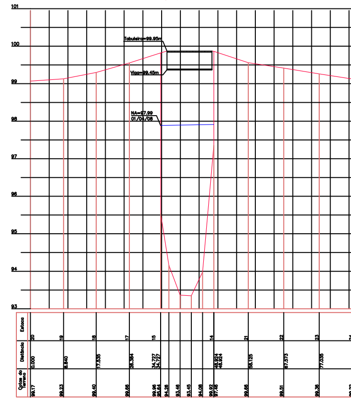
Perfil Longitudinal - Ponte 01 Igarapé Altamira
