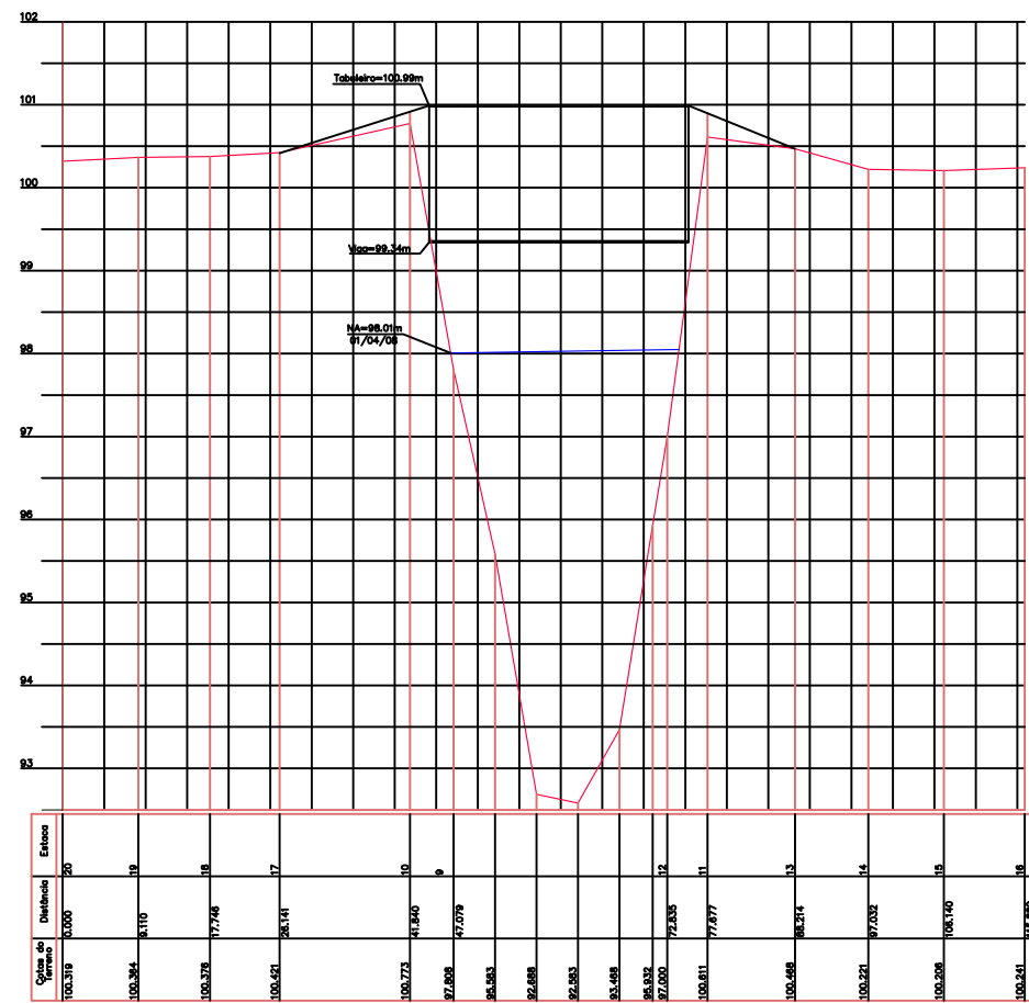
Perfil Longitudinal - Ponte 07 Igarapé Panelas
