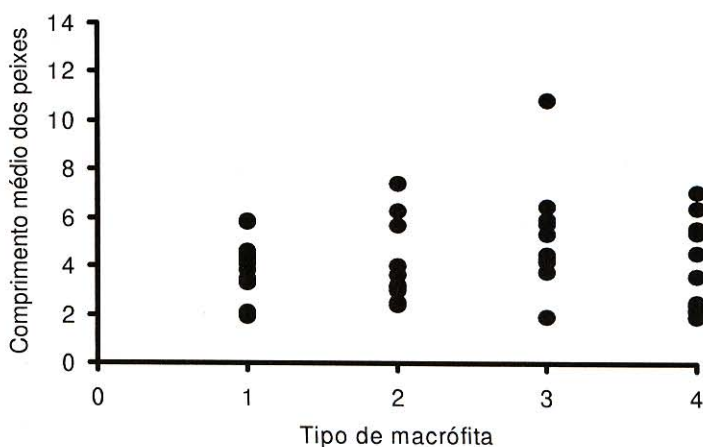
Figura 2. Comprimento (cm) médio dos peixes em cada amostra por tipo de macrófita: 1- "capim morto", 2- Eichhornia spp., 3- E. polystachya e 4- P. repens (ANOVA: F= 1,763 ; p= 0,17 ).
