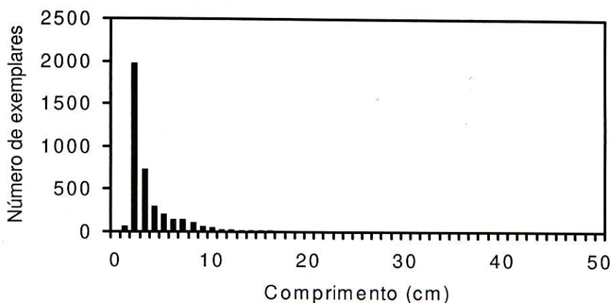
Figura 1. Distribuição das classes de tamanho (Ls) da ictiofauna associada às raízes de macrófitas.
