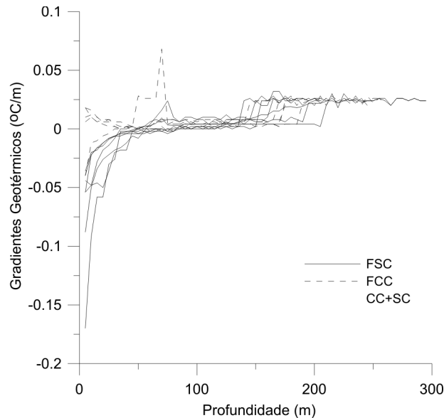
Figura 3 - Gradientes geotérmicos da região de Manaus (AM). FSC – furo sem cobertura, FCC – furo com cobertura, CC + SC – média de todos os furos.
