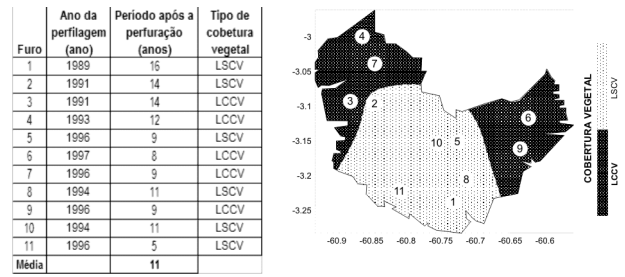
Figura 1 - Localização dos gerfis geotérmicos em Manaus – AM.
